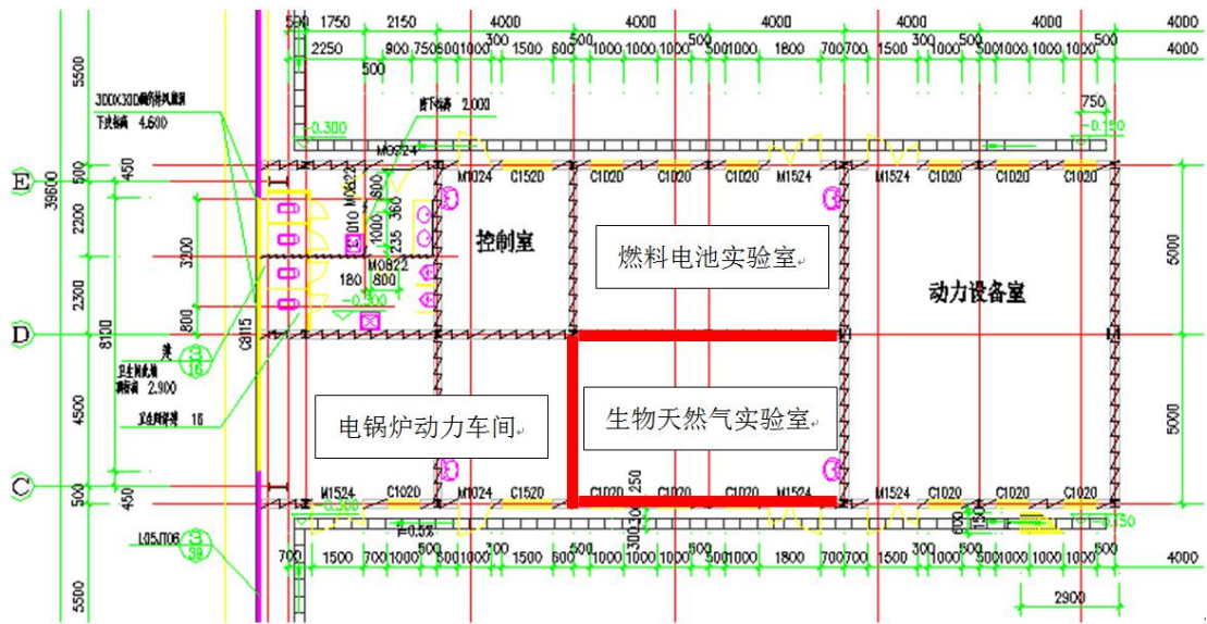
图 2 一层待拆除墙壁
